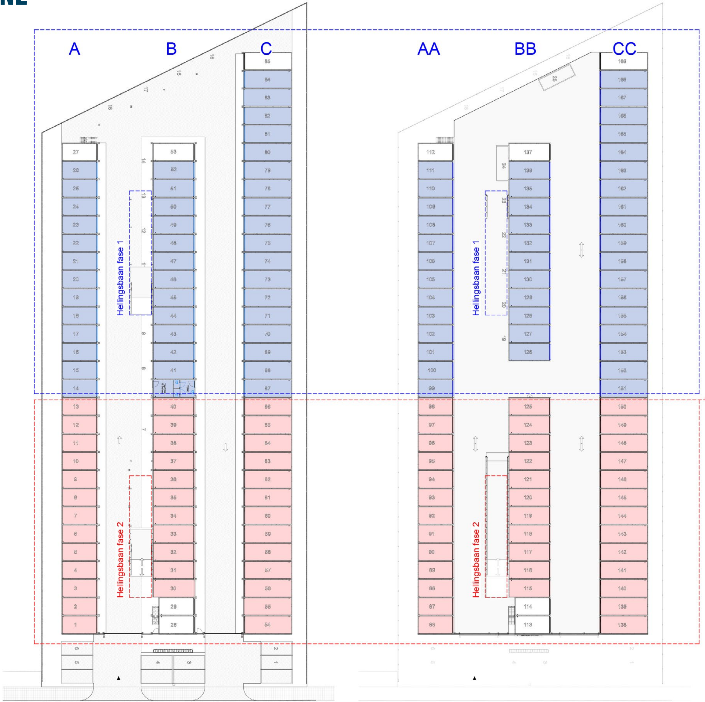
Begane grond
